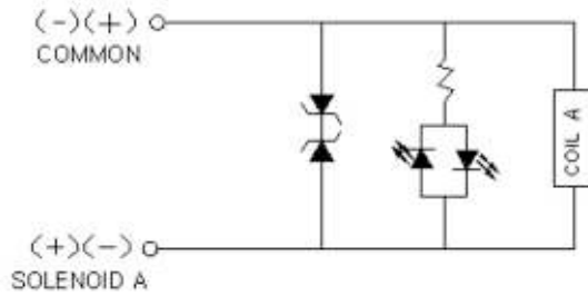
<Single Circuits>
