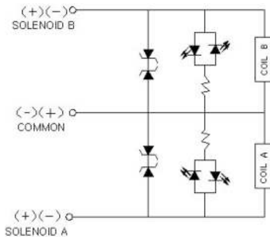
<Double Circuits>
